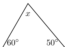
A) Triángulo 1
